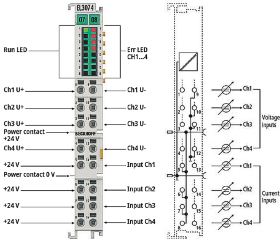
Fig. 52: EL3074
