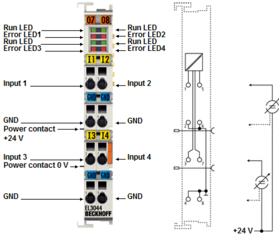
Fig. 28: EL3044
